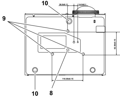
底視圖
